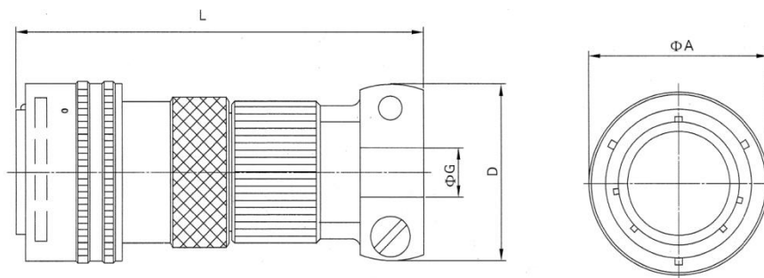
Straight plug (MS3116J)
