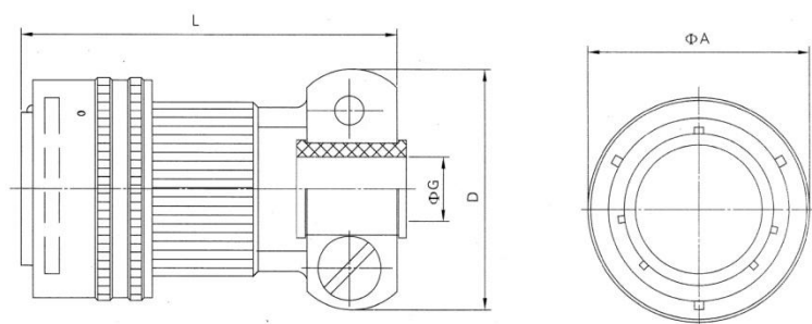
Straight plug (MS3116F)
