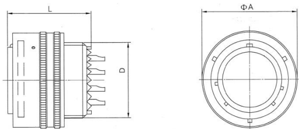
Straight plug (MS3116R)
