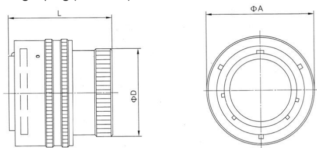
Straight plug (MS3116E)
